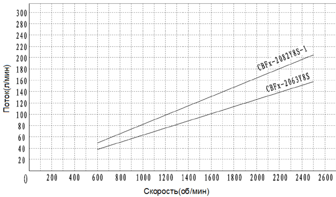
Диаграмма Поток/Скорость
